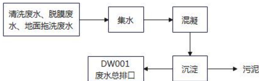
图 4-1 废水治理工艺流程图
