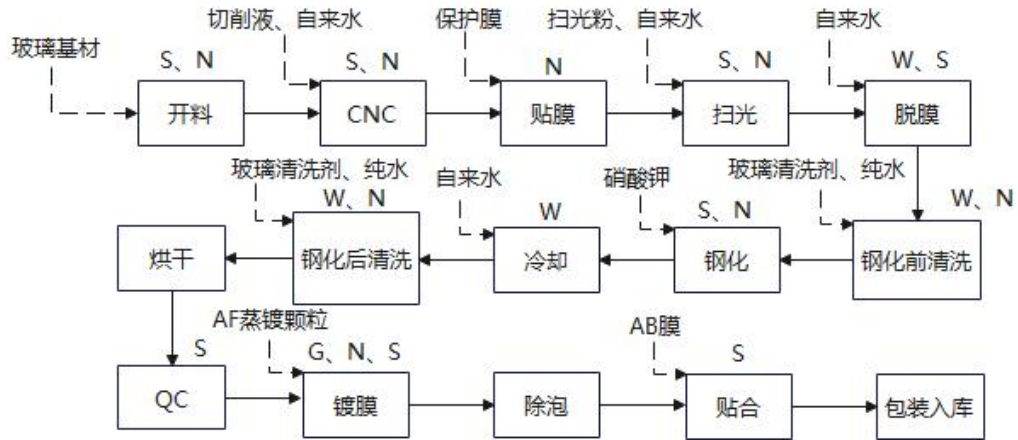
图 2-2 钢化玻璃膜生产工艺流程及产污节点图
